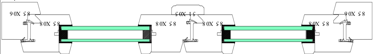
Coupe horizontale. Echelle 1/3
