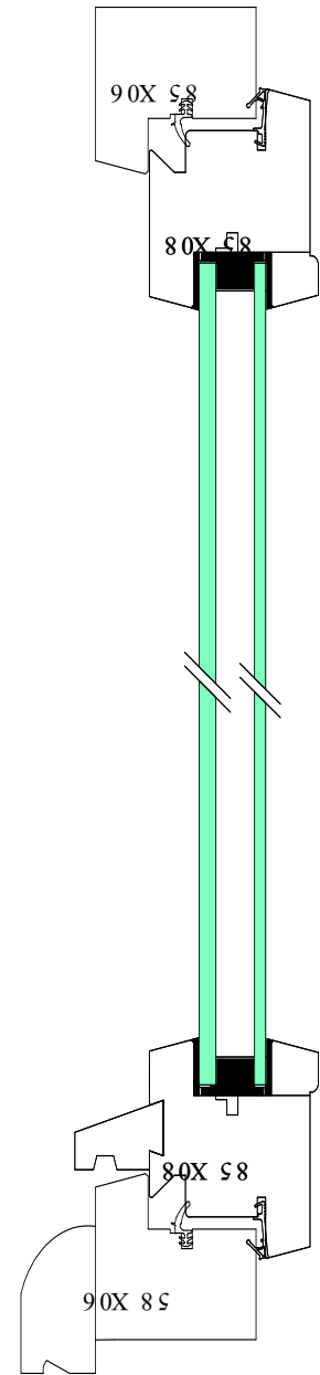
Coupe verticale. Echelle 1/3
